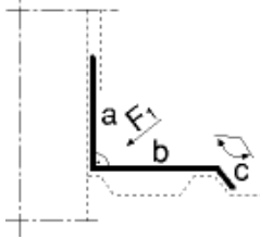
Anschlußprofil f. Attika/Ortgang 1
