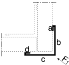
Außeneckprofil
