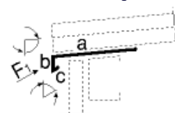
Rinneneinhangblech
