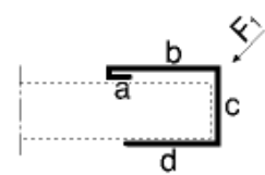
seitliches Einfaßprofil
