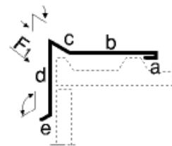
Ortgangprofil 3
