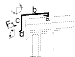
Sichtschutzprofil
